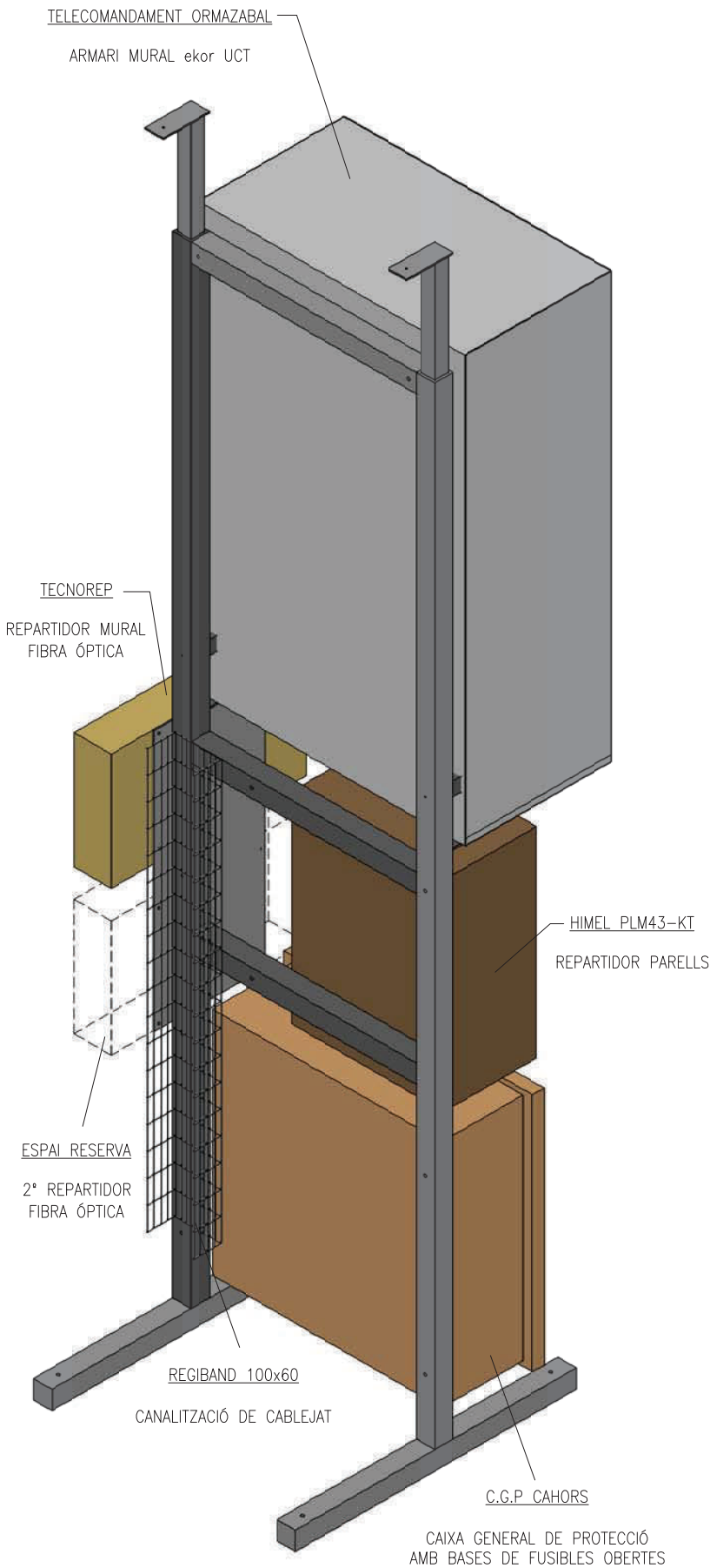
VISTA GENERAL ISOMÉTRICA 2 AMB INSTAL·LACIÓ
