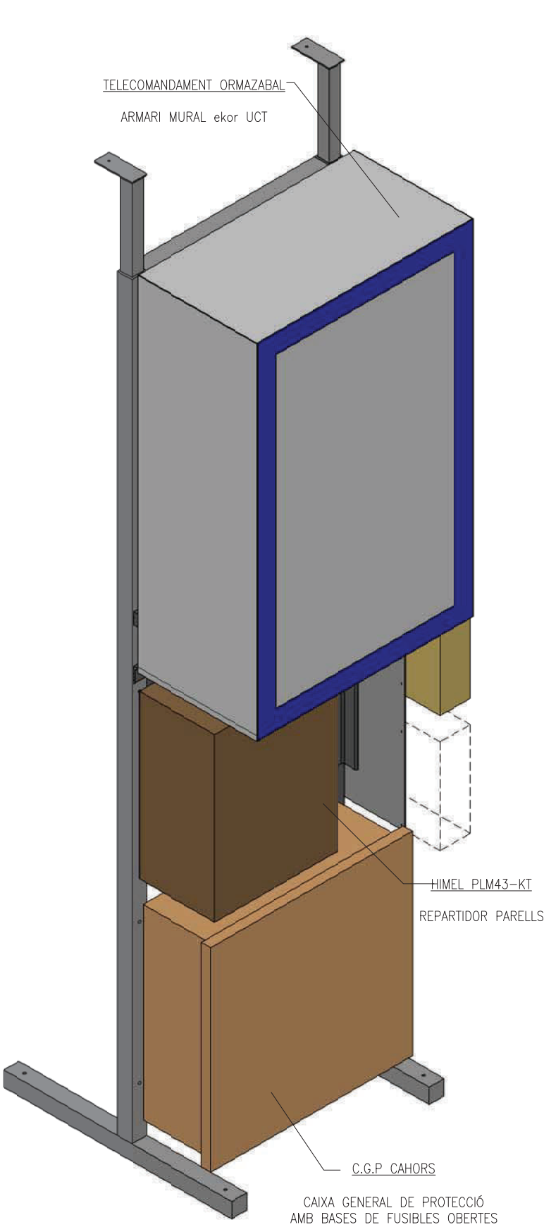
VISTA GENERAL ISOMÉTRICA 1 AMB INSTAL·LACIÓ
