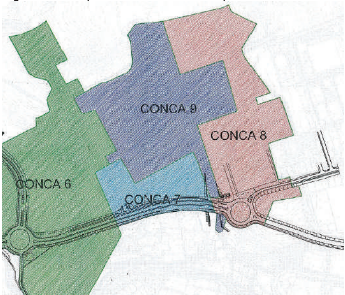
Figura 3: Conques de l'As-Built de l'Apliació de la Carretera BP-1413
