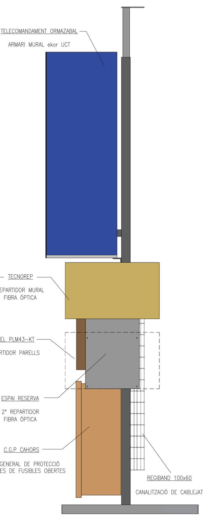
VISTA GENERAL PERFIL LATERAL AMB INSTAL·LACIÓ
