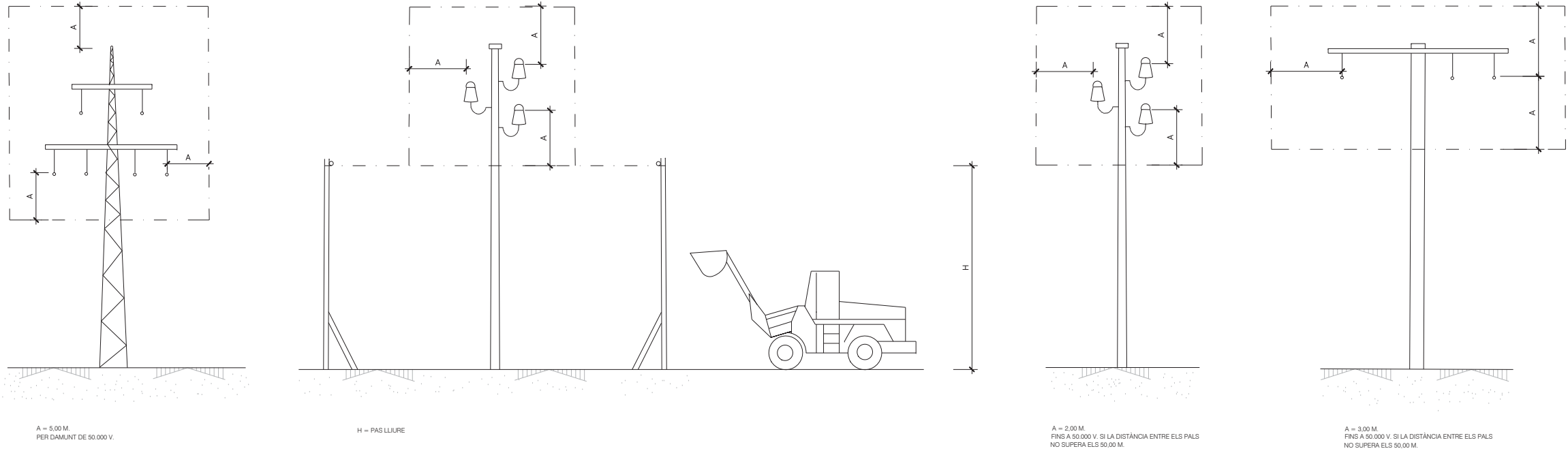
LÍNIES ELÈCTRIQUES AÈRIES
