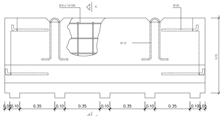
SECCIÓ A-A'
