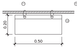
DETALL 2
