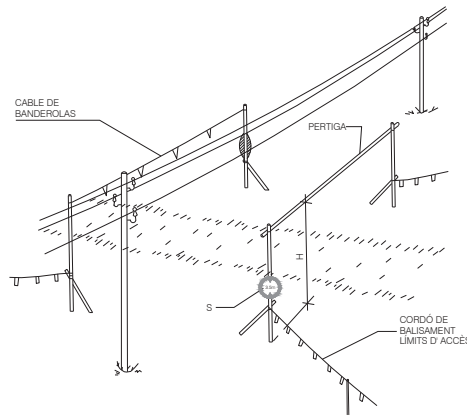
DETALL 2
