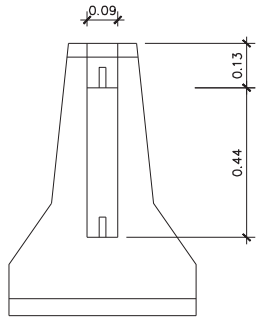
ALÇAT TRANSVERSAL
