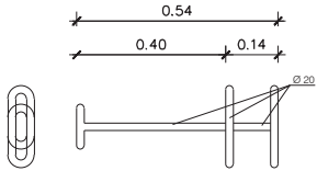
CLAVILLA D'UNIÓ
