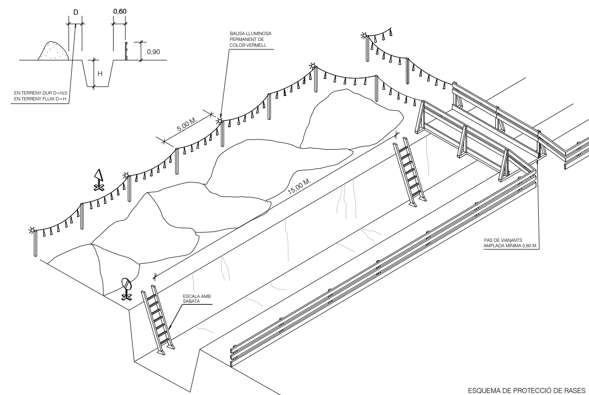
ESQUEMA DE PROTECCIÓ DE RASES ESCALA S/E
