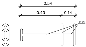
CLAVILLA D'UNIÓ
